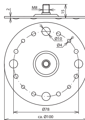
Maßbild
