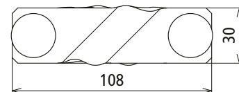
Maßbild
