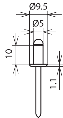
Maßbild
