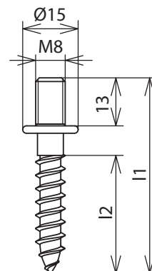
Maßbild
