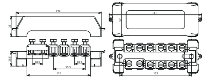
Maßbild
