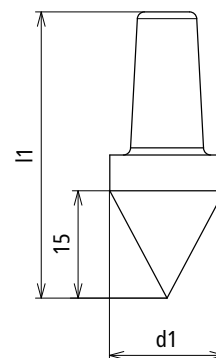
Maßbild
