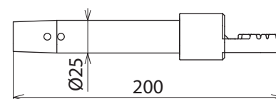
Maßbild
