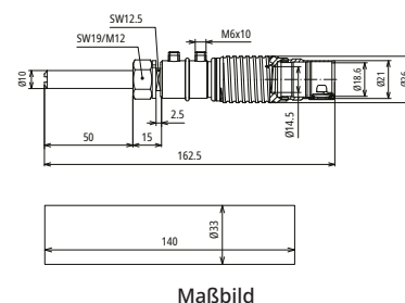
Maßbild
