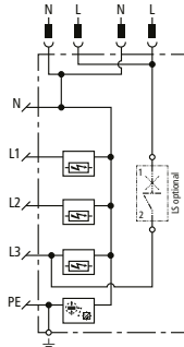
Prinzipschaltbild
