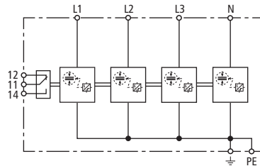
Prinzipschaltbild
