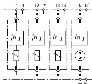
Prinzipschaltbild
