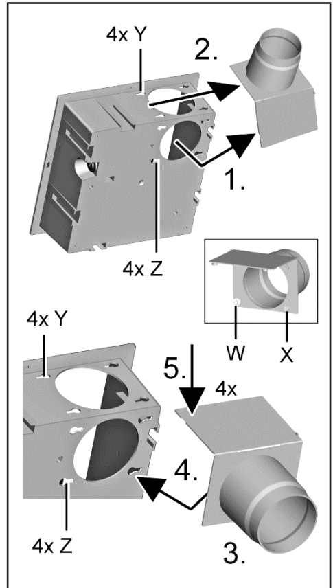
Kunststoff-Verschlussklappe vorbereiten: Ausblas nach oben, links oder rechts
