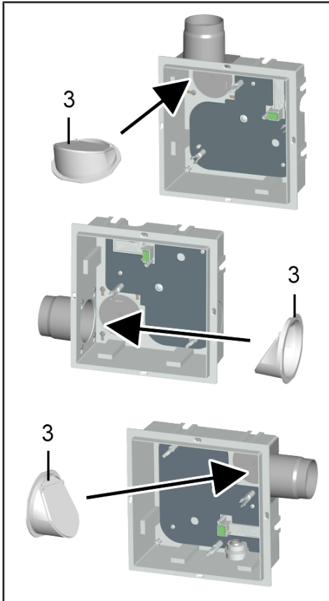
Kunststoff-Verschlussklappe vorbereiten: Ausblas nach oben, links oder rechts
