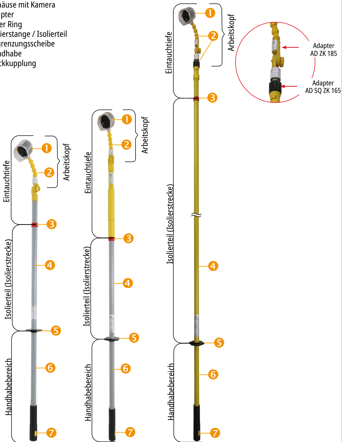
Bild 10 Isolierstangen mit Arbeitskopf
