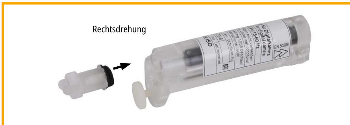
Bild 4 Flügelerschraube mit Bajonettverschluss
